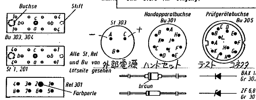
FSE-38/58 内部接続図
